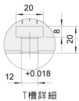
T槽詳細
