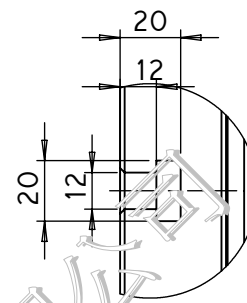
細部放大圖 L 比例 2:5
