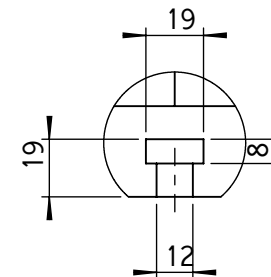
T溝 細部放大圖 T 比例 2 : 5
